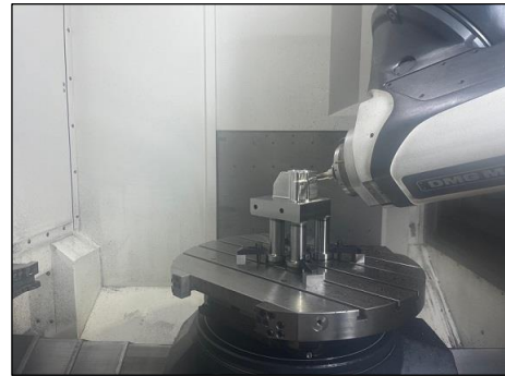
切削加工
