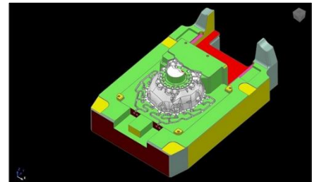
3D 設計イメージ
