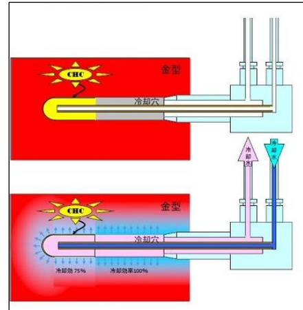
『CHC』の仕組み(同社 HP より)
