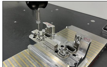
金型検査
